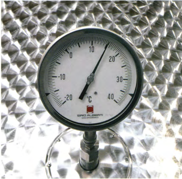
TERMOMETRO IN ACCIAIO INOX A GAS INERTE PRECISIONE +/- 1% BULBO DI IMMERSIONE L.600mm THERMOMETER STAINLESS STEEL THERMOMETER WITH INERT GAS PRECISION +/- 1% - IMMERSION BULB LENGTH 600mm
