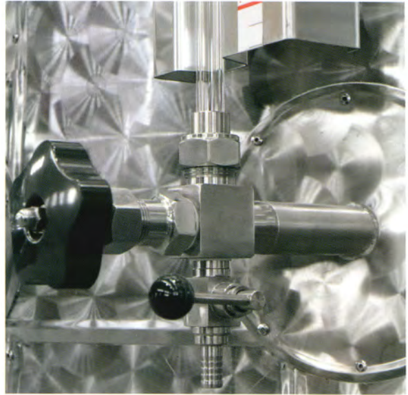
INDICATORE LIVELLO CON RUBINETTI A SPILLO E TUBO IN VETRO CERTIFICATO LEVEL INDICATOR WITH CORE VALVE AND CERTIFICATE GLASS TUBE
