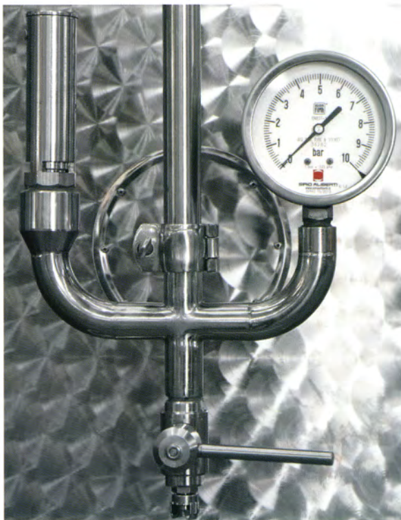
GRUPPO ARIA IN ACCIAIO INOX CON MANOMETRO PRECISIONE +/- 1% E VALVOLA DI SICUREZZA PRESSURE PIPE-LINE WITH MANOMETER PRECISION +/- 1% AND STAINLESS STEEL SAFETY VALVE
